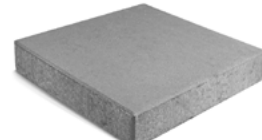
Hansa 8 Plus 500 × 500 × 80 mm
