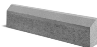
Veja 5×20 1000 × 50 × 200 mm
